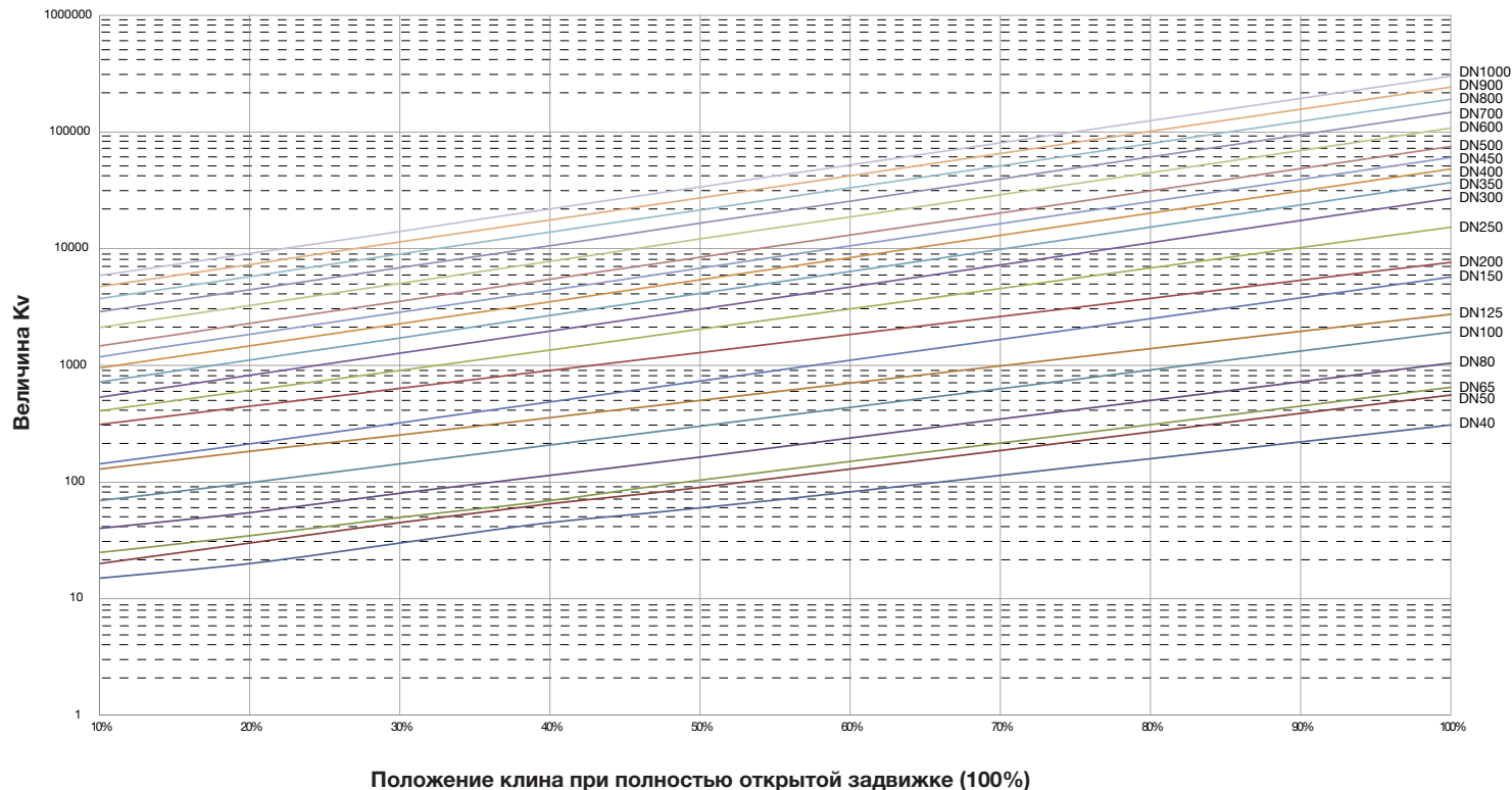
Величины Kv для клиновых задвижек диаметрами DN40 – DN1000
