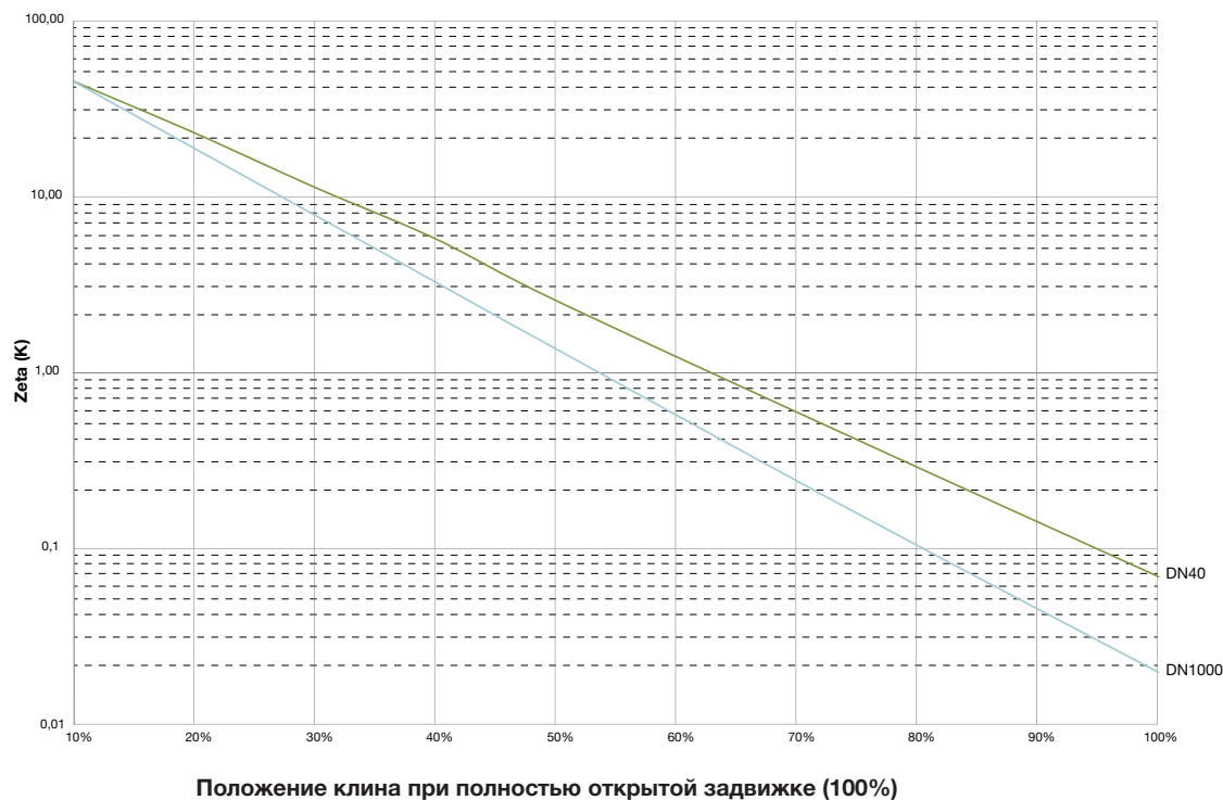
Значения ZETA (K) для клиновых задвижек диаметрами DN40 – DN1000
